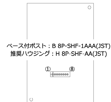
背面図
