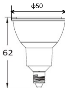
<外形寸法図>
